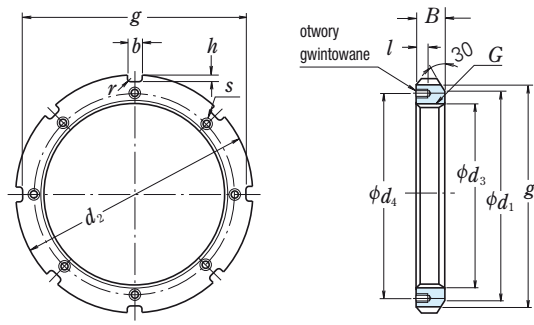
Nakrętka z podkładką kształtową
