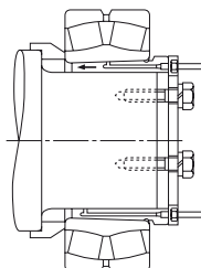
Rys. 14.7 Osadzanie łożysk z tuleją specjalną i prasą hydrauliczną
