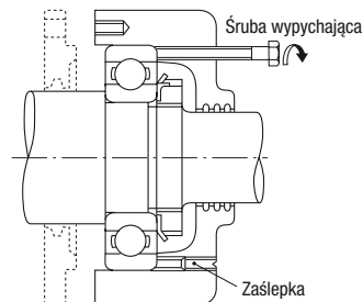
Rys. 14.10 Zdejmowanie pierścienia zewnętrznego przy użyciu śrub wypychających
