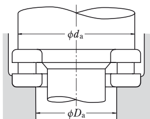
Rys. 11.4 Średnice powierzchni podpartej dla łożysk wałeczkowych wzdłużnych
