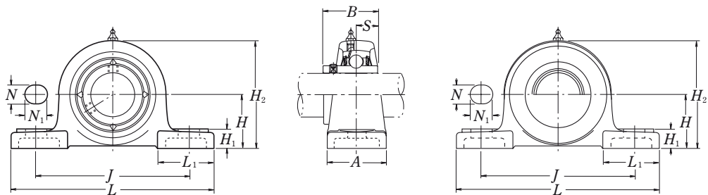
Typ z pokrywą przeciwpływową tłoczoną blaszaną przelotowa Z-UCP...D1 nieprzelotowa ZM-UCP...D1
