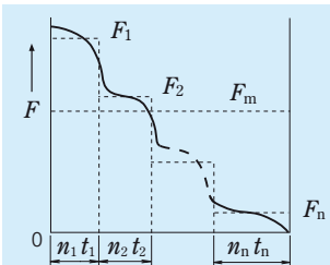
Rys. 5.7 Przyrostowa zmiana obciążenia
