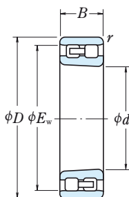
NN Otwór stożkowy
