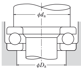
Rys. 11.3 Średnice powierzchni podpartej dla łożysk kulkowych wzdłużnych
