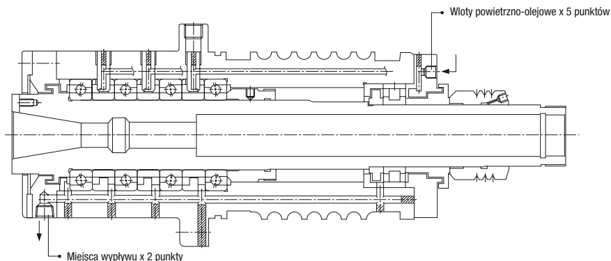
Rys. 12.10 Smarowanie olejowo-powietrzne
