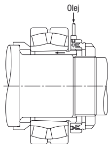
Rys. 14.6 Osadzanie łożyska za pomocą nakrętki hydraulicznej
