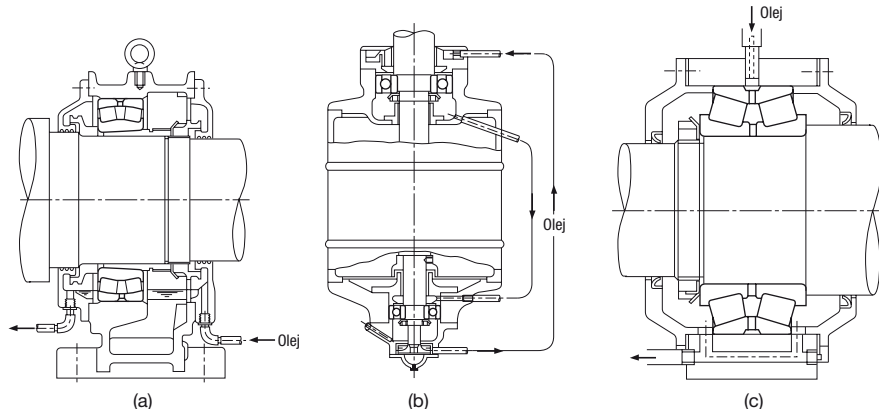
Rys.12.7 Smarowanie obiegowe
