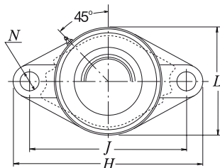
Typ z pokrywą przeciwpylową tłoczoną blaszaną przelotowa Z-UCFL...D1 nieprzelotowa ZM-UCFL...D1
