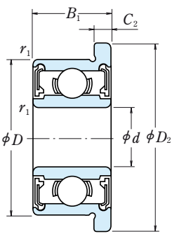
Typ z uszczelkami bezszykowymi VV
