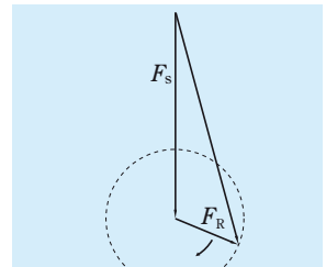
Rys. 5.10 Obciążenie wirujące i obciążenie stacjonarne
