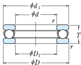
Z płaskim pierścieniem zewnętrznym
